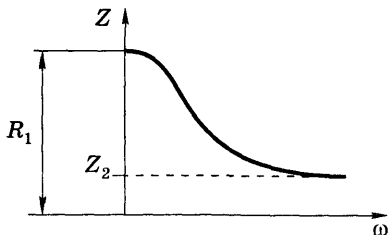
Рис. 14.11. Типичная зависимость импеданса живой ткани от частоты
