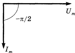
Рис. 14.7. Векторная диаграмма при ин- дуктивной нагрузке
