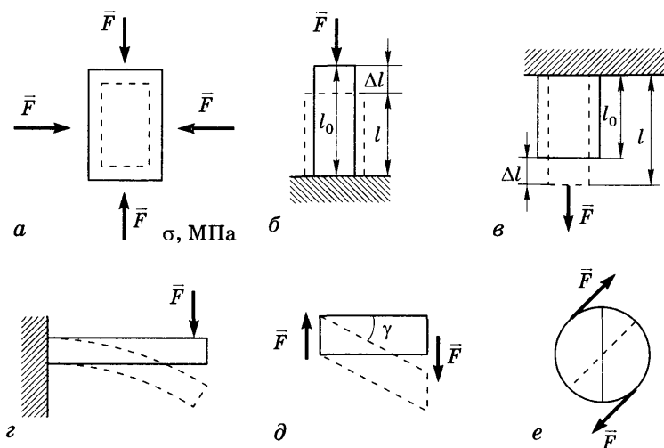
Рис. 5.4. Основные виды деформации твердых тел: а — всестороннее сжатие; б — одноосное сжатие; в — одноосное растяжение; г — изгиб; д — сдвиг; е — кручение
