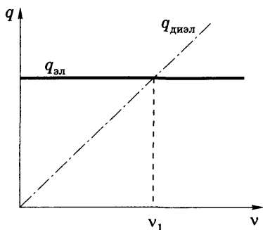
Рис. 17.4. Частотная зависимость тепловой мощности, выделяющейся под действием УВЧ-поля в электролите и диэлектрике
