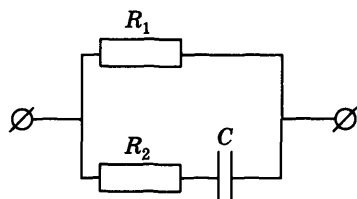
Рис. 14.12. Эквивалентная электрическая схема живой ткани
