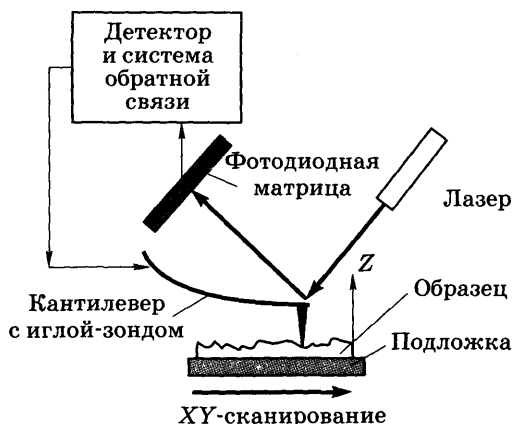
Рис. 25.7. Принципиальная схема АСМ
