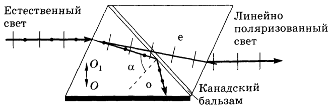
Рис. 19.6. Призма Николя: обыкновенный луч o испытывает полное отражение от склейки, а необыкновенный луч e проходит через нее и выходит из призмы
