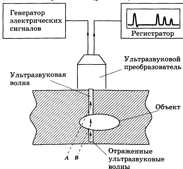
Рис. 7.9. Принципиальная схема эхолокации в А-режиме
