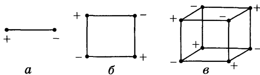
Рис. 12.5. Электрически нейтральные мультиполи: а — диполь; б — квадруполь; в — октуполь
