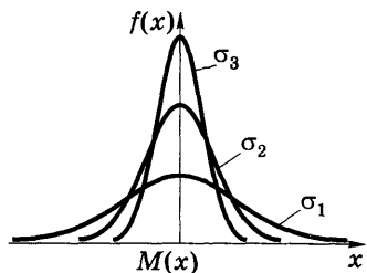
Рис. 3.6. Вид кривой нормального распределения при разных значениях \sigma ( \sigma_3 < \sigma_2 < \sigma_1 )
