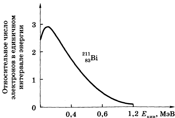
Рис. 28.2. Энергетический спектр \beta -частиц при распаде {}_{83}^{211}\text{Bi}
