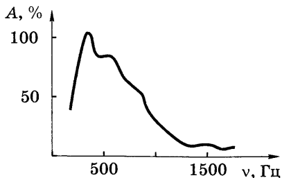
Рис. 7.2. Спектр шума
