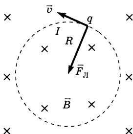
Рис. 15.5. Движение заряда в однородном магнитном поле, где \vec{v} \perp \vec{B}
