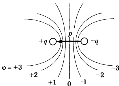
Рис. 12.3. Поле диполя. Линии равного потенциала электрического поля диполя
