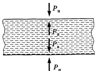
Рис. 9.20. Трансмуральное давление
