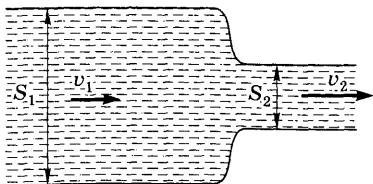
Рис. 9.3. Условие неразрывности струи
