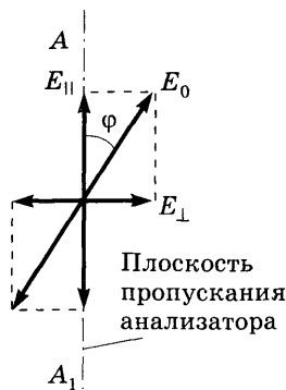
Рис. 19.8. К выводу закона Малюса
