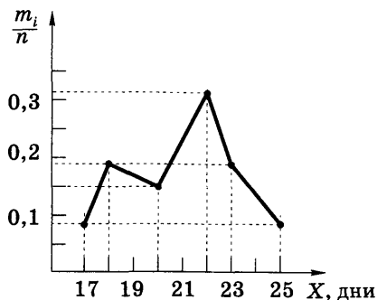
Рис. 4.2. Полигон относительных частот
