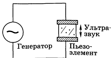
Рис. 7.8. Обратный пьезоэффект
