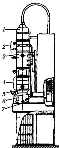
Рис. 25.6. Упрощенная схема (а) и внешний вид (б) просвечивающего электронного микроскопа (ПЭМ):
