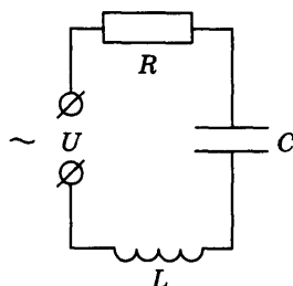
Рис. 14.8. Омическая, емкостная и индуктивная нагрузки в цепи переменного тока
