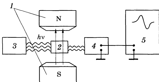
Рис. 26.2. Схема установки для наблюдения ЭПР:
