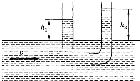
Рис. 9.5. Метод определения скорости движения жидкости
