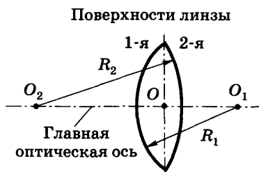
Рис. 25.1. Схема двояково-выпуклой линзы
