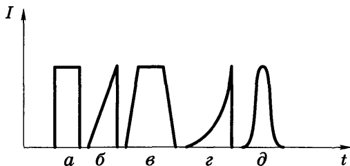
Рис. 16.4. Некоторые виды импульсных токов:
