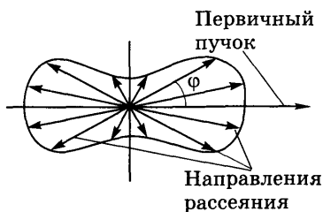
Рис. 21.4. Индикатриса молекулярного рассеяния света
