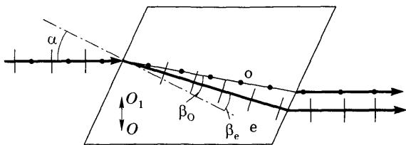
Рис. 19.5. Двулучепреломление света в кристалле: O_1O — направление оптической оси кристалла; о — обыкновенный луч; е — необыкновенный луч
