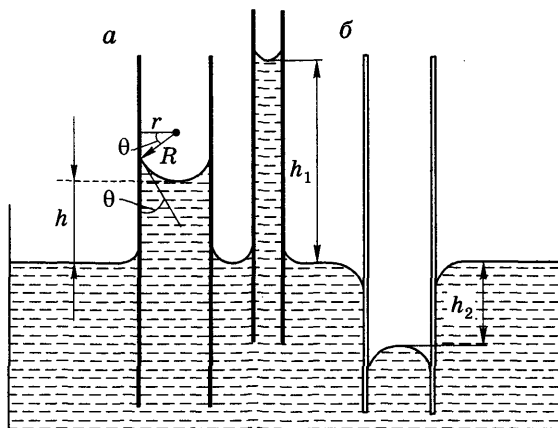
Рис. 8.5. Капиллярные явления:
