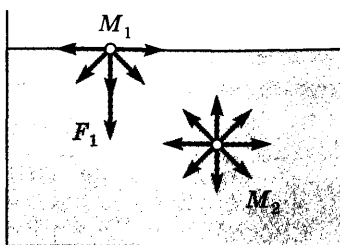
Рис. 8.1. Молекулярные силы, действующие на молекулу M_1 поверхностного слоя и молекулу M_2 внутри объема
