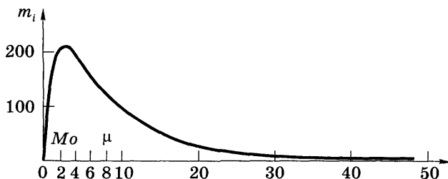
Рис. 4.4. Зависимость частоты заболевания от возраста
