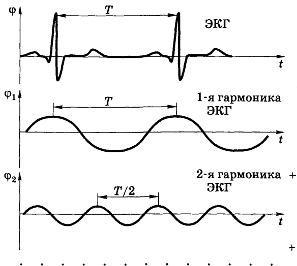
Рис. 6.7. Разложение ЭКГ на отдельные гармонические составляющие
