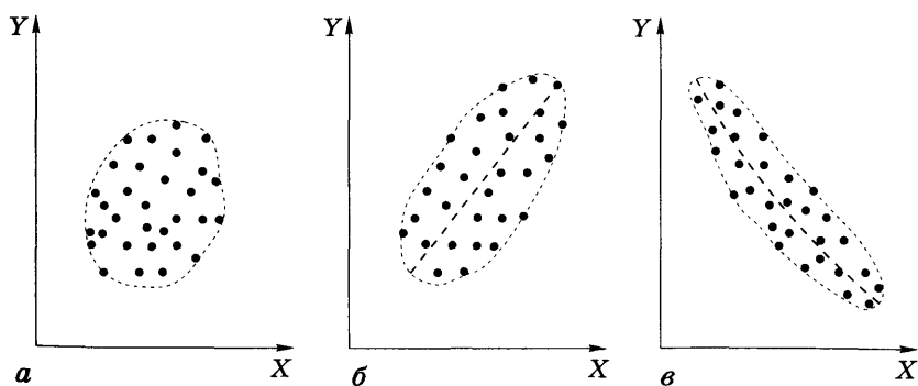
Рис. 4.5. Соответствие формы корреляционного поля степени корреляционной связи между величинами X и Y :
