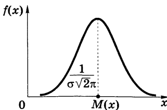
Рис. 3.5. Вид кривой нормального распределения случайной величины X
